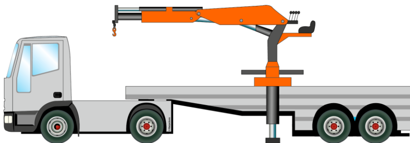
Grue de chargement montée en position centrale
